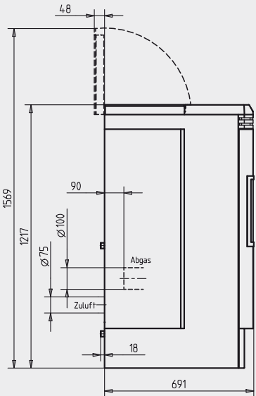
Seitenansicht
