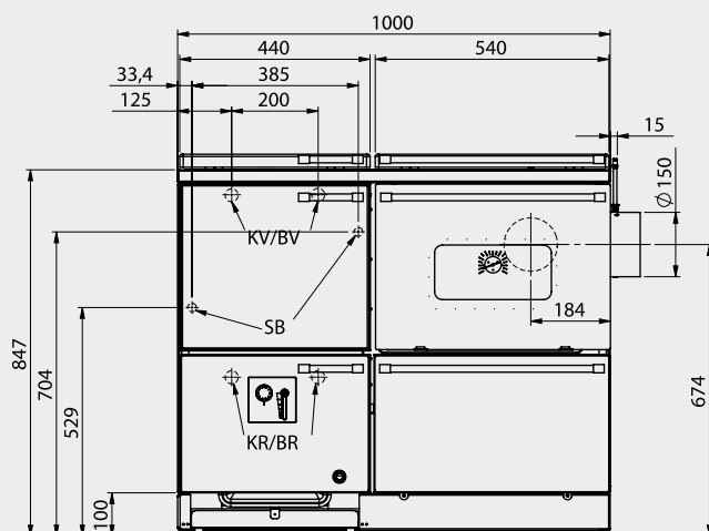
VestowIN Premium 202 – Vista frontale
