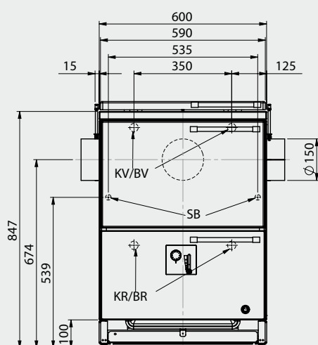
VestowIN Klassik 220 – Vista frontale
