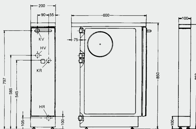
Modulo porta accessori Vesto 200
