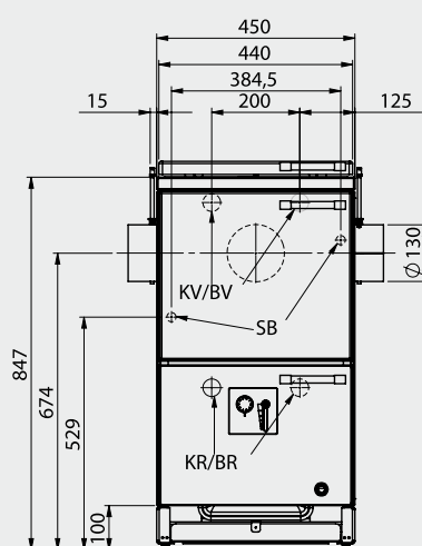
VestowIN Klassik 170 – Vista frontale
