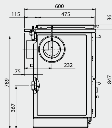
VestowIN Klassik 220/170 – Vista laterale
