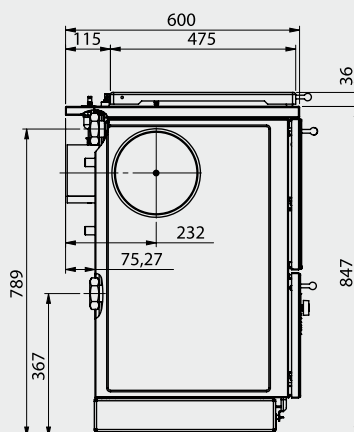
VestowIN Premium 202 – Vista laterale
